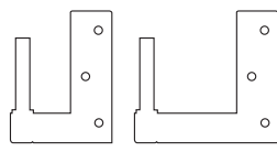
Jamb Pintel Offset - 1", 2"
